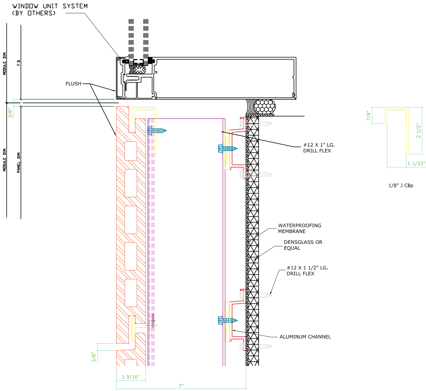
E WINDOW SILL Lrg Scale: 3 3/4"=1'
