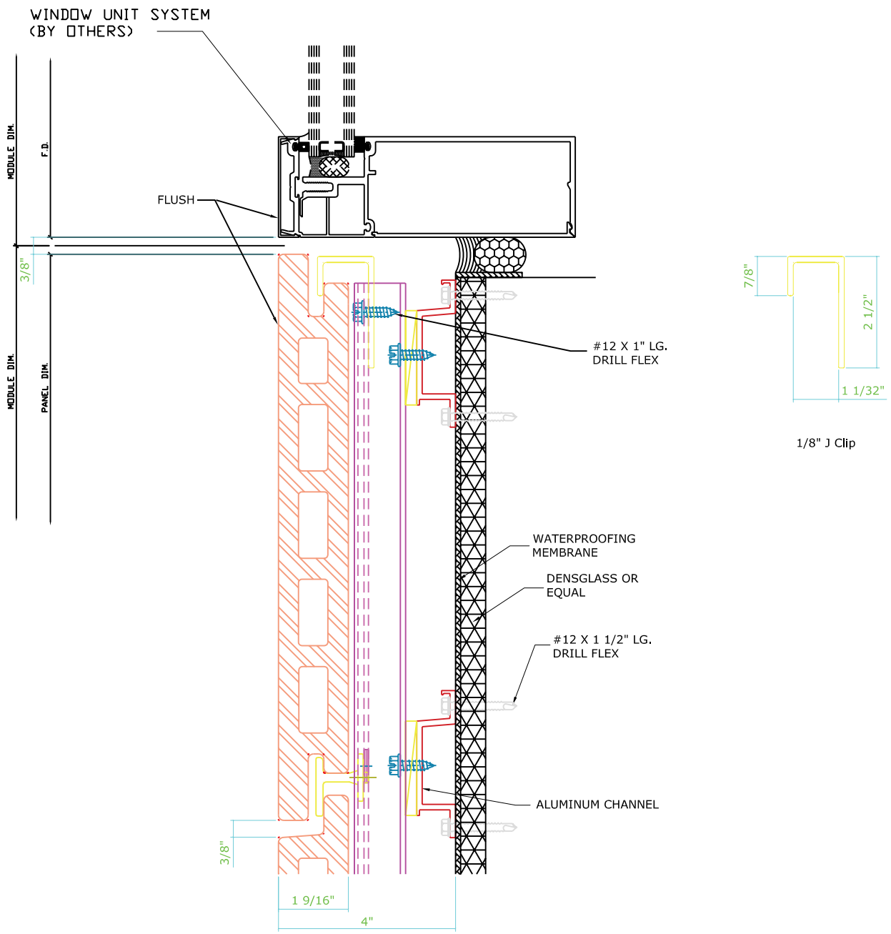
E WINDOW SILL Lrg Scale: 3 3/4"=1'
