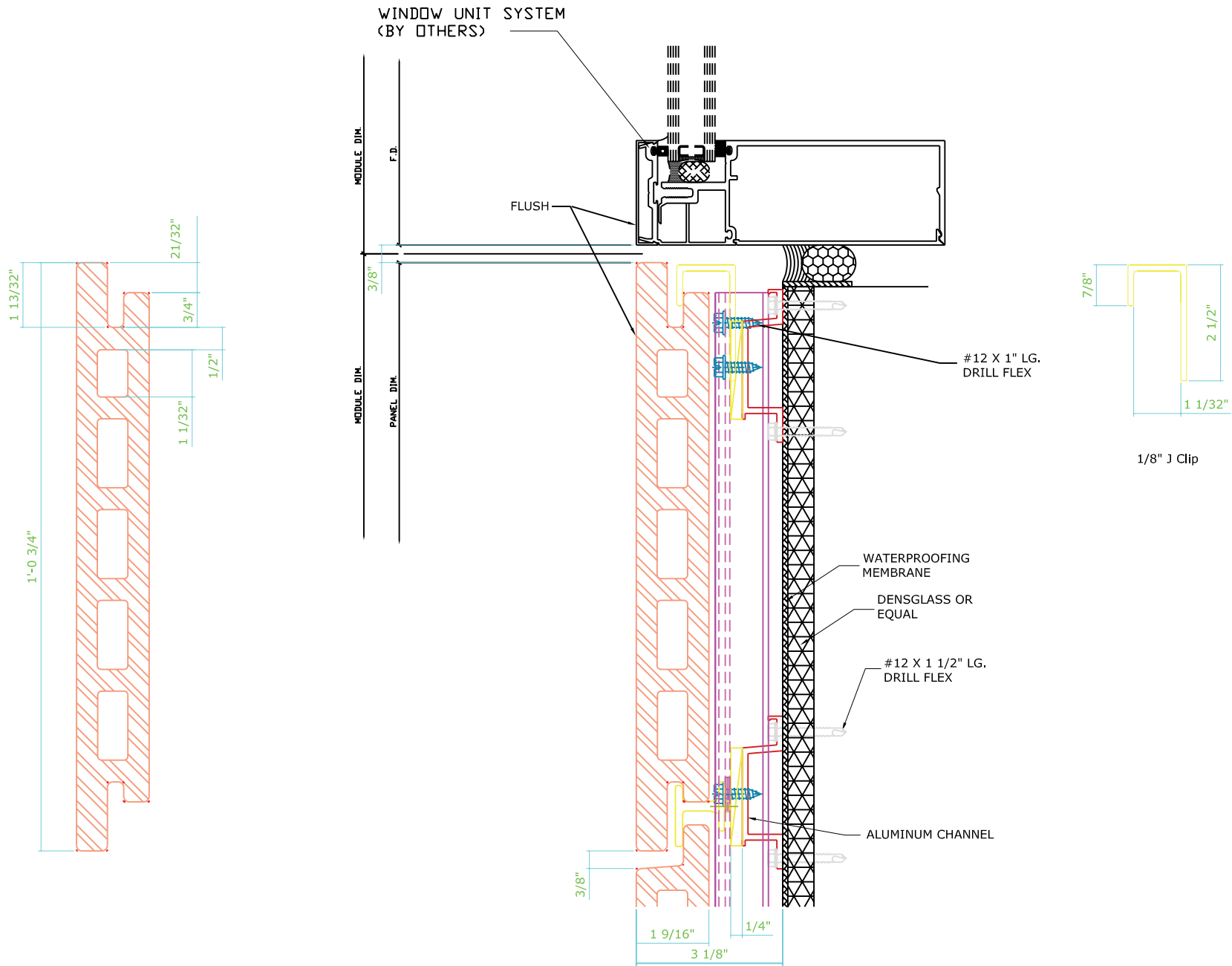
E WINDOW SILL Lrg Scale: 3 3/4"=1'
